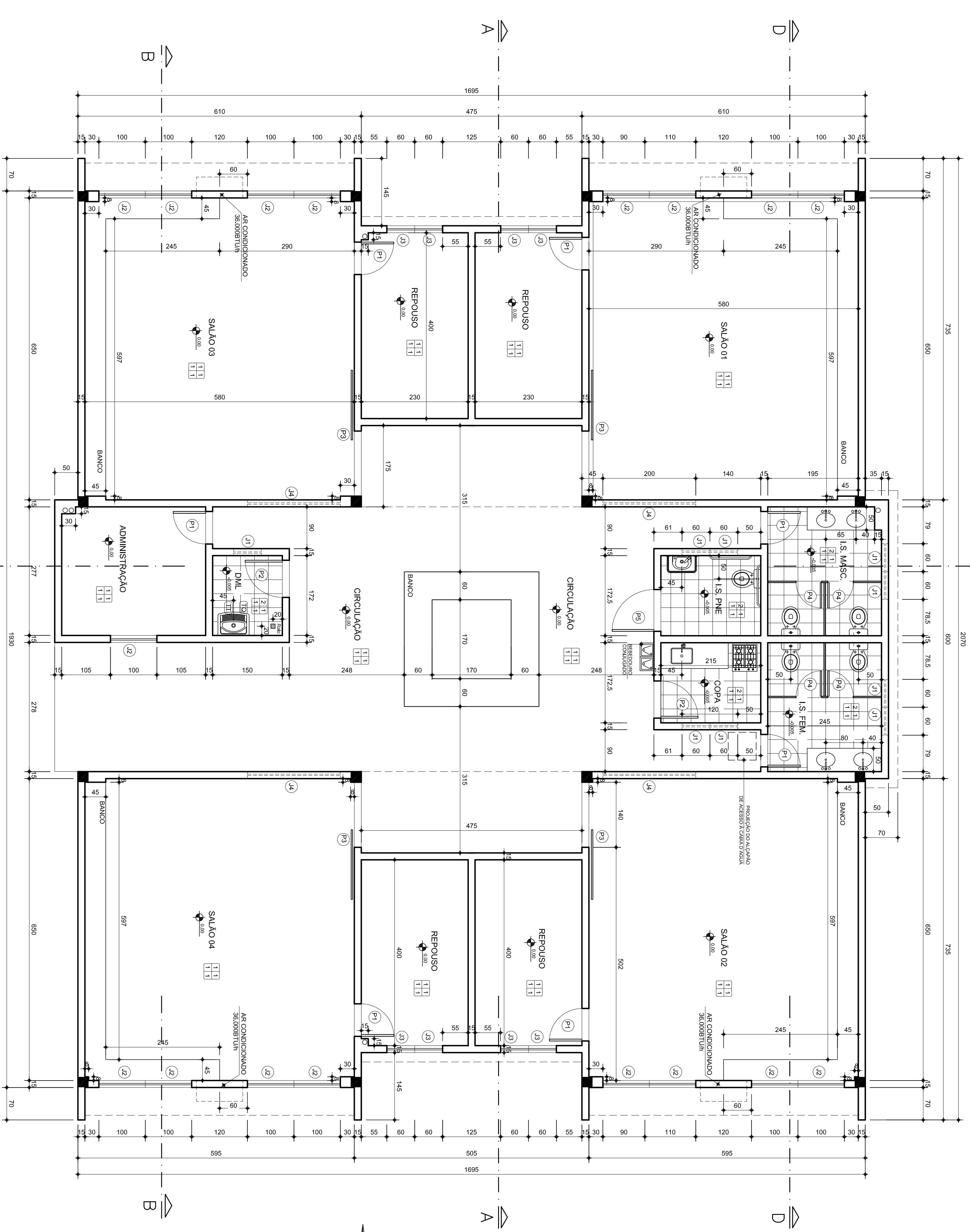
PLANTA BAIXA Escola 1/50
